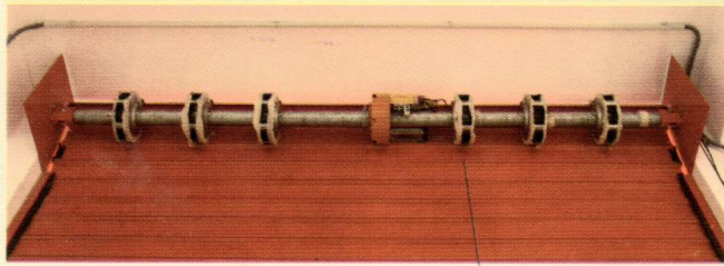
Άξονας ρολού γκαραζόπορτας με βιομηχανικό τύπου μοτέρ (Φ88).
